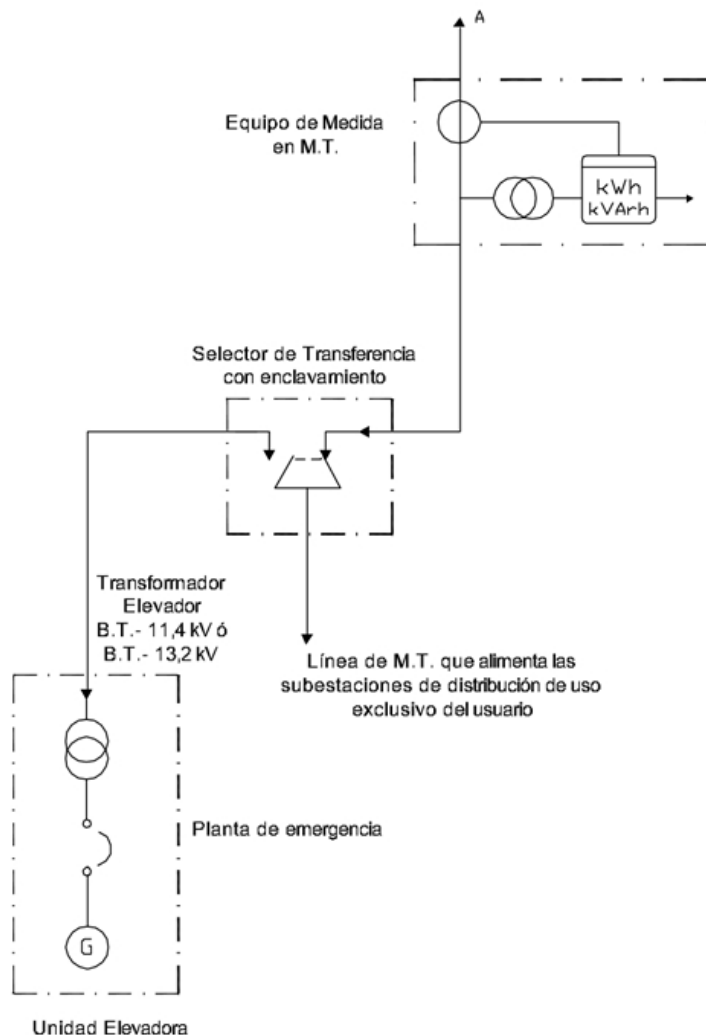
ACOMETIDA DESDE RED SUBTERRÁNEA DE M.T.
