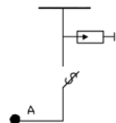
FORMAS DE ALIMENTACIÓN DESDE EL SISTEMA DE DISTRIBUCIÓN DE CODENSA ACOMETIDA DESDE RED ÁEREA DE M.T.
