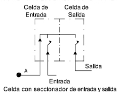
ACOMETIDA DESDE RED SUBTERRÁNEA DE M.T.
