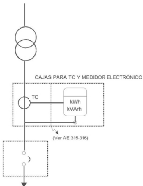
FIG 1 -CAJAS PARA MEDICIÓN SEMIDIRECTA
