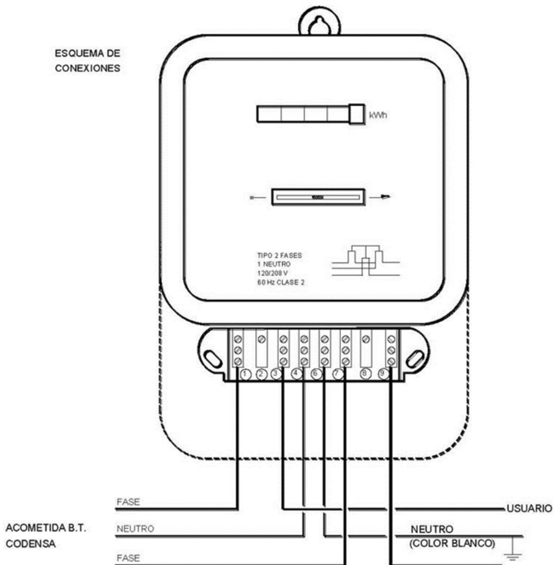
ESQUEMA ELÉCTRICO
