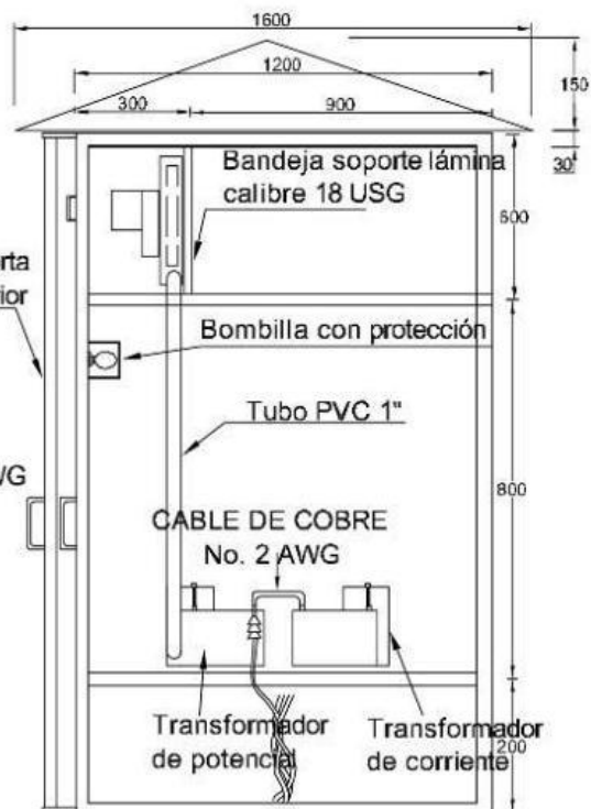
VISTA LATERAL
