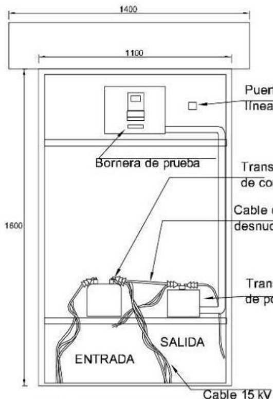
VISTA FRONTAL SIN PUERTA
