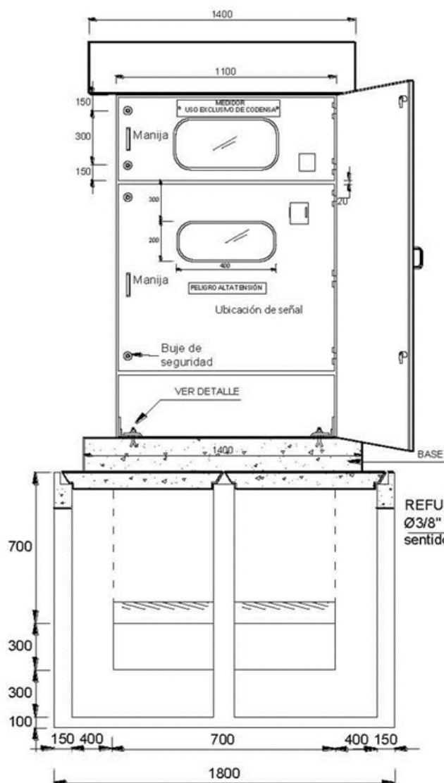
CORTE B-B
