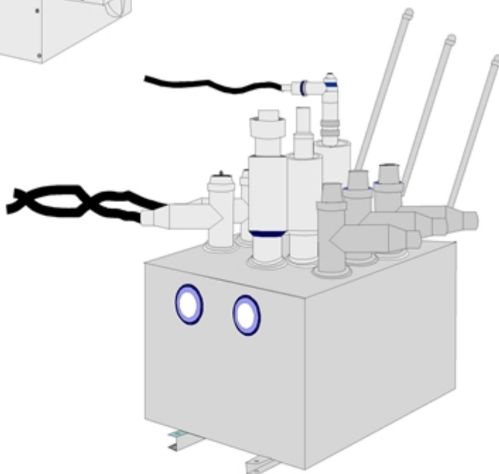
SECCIONADORES DE MANIOBRA TIPO VAULT SUBSURFACE SUBMERSIBLE
