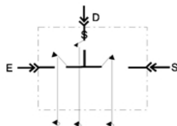
INSTALACIÓN TIPO CELDA CON PROTECCIÓN
