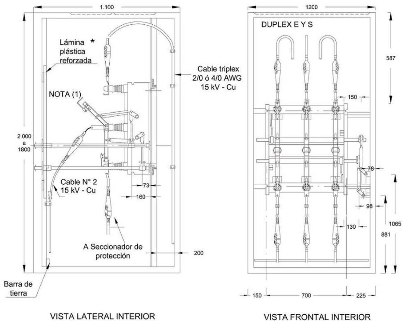
FIGURA 1 CELDA DUPLEX PARA MT (VISTA INTERNA FRONTAL Y LATERAL)
