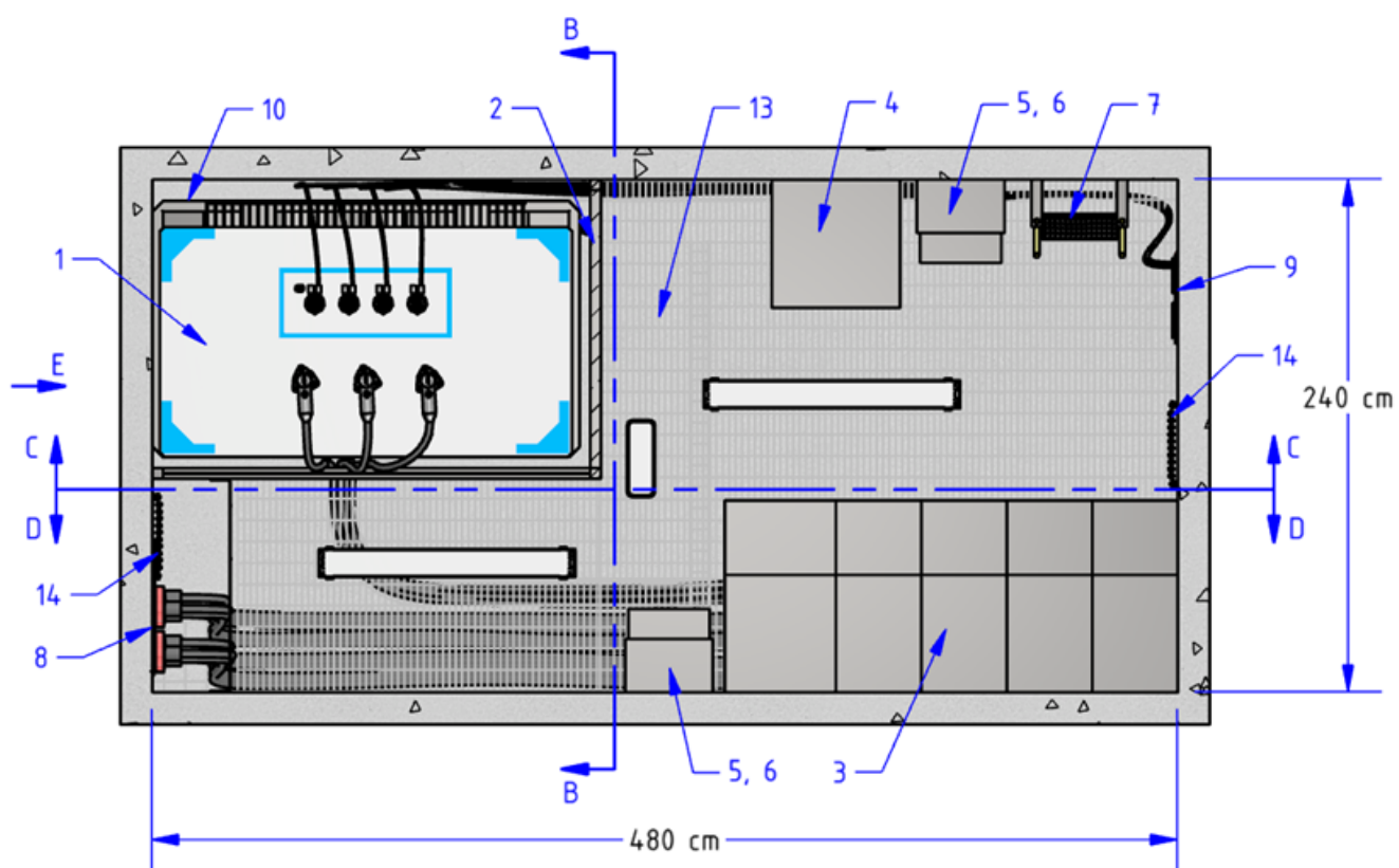
Figura No 1 Vista planta
