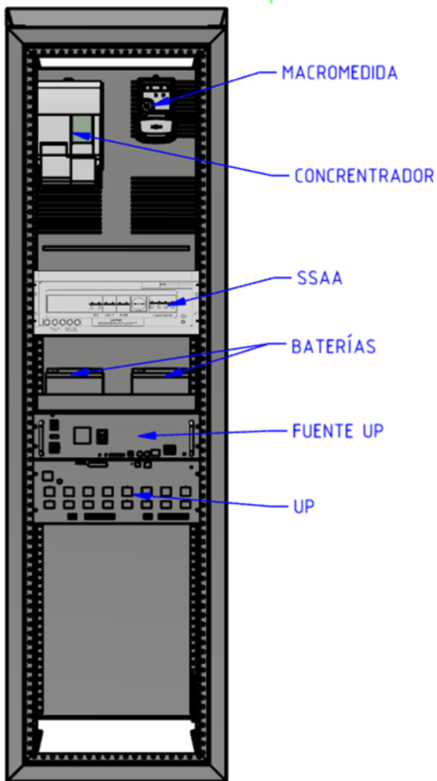
Figura No 7 Tablero TLC.
