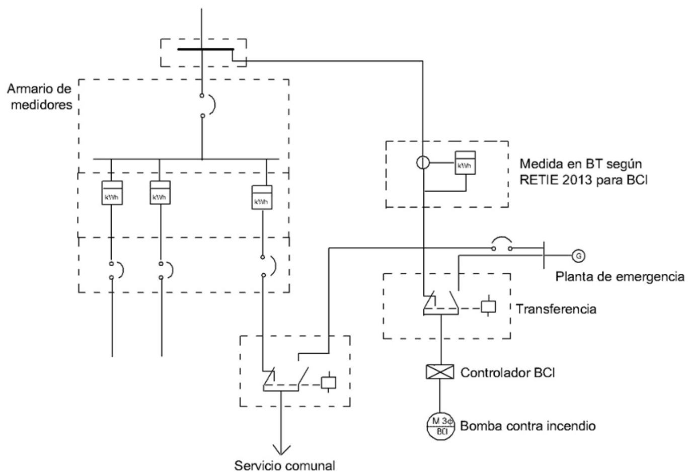
Figura 3. Acometida con servicio normal y de emergencia
