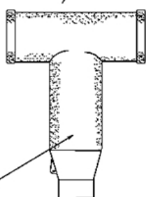
Terminal tipo T 600 A (Norma CS 336)
