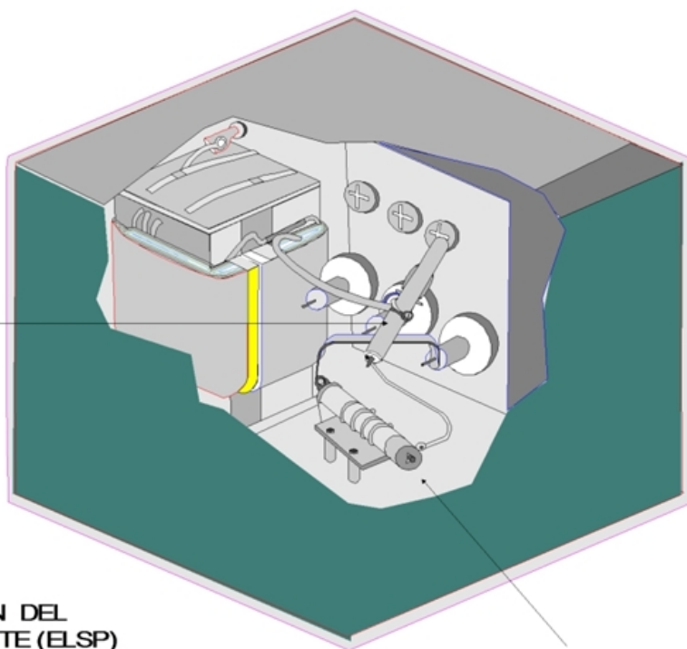
Fusible limitador de corriente
