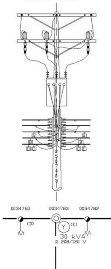
CIRCUITO AÉREOS
