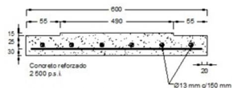
CORTE C - C'
