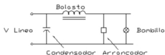
Disposición Bolasto reactor para luz de sodio
