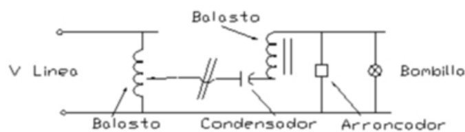
Disposición Bolasto CWA (Autoregulado) para luz de sodio
