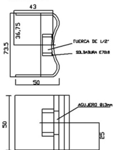
SOPORTE BRAZO LUMINARIA PLATINA DE 3/16" DE ESPESOR
