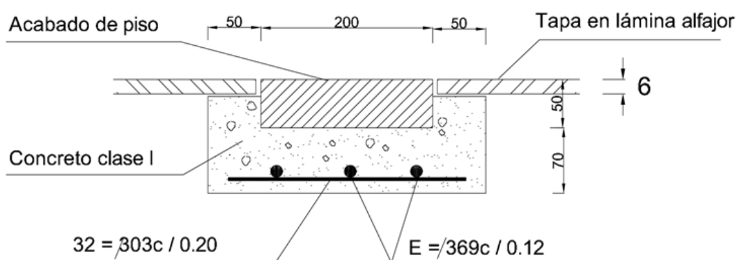
DETALLE 2
