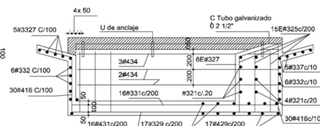
REFUERZO CORTE B-B Esc: Sin
