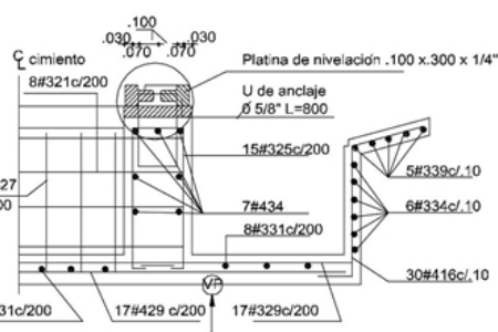
REFUERZO CORTE A-A
