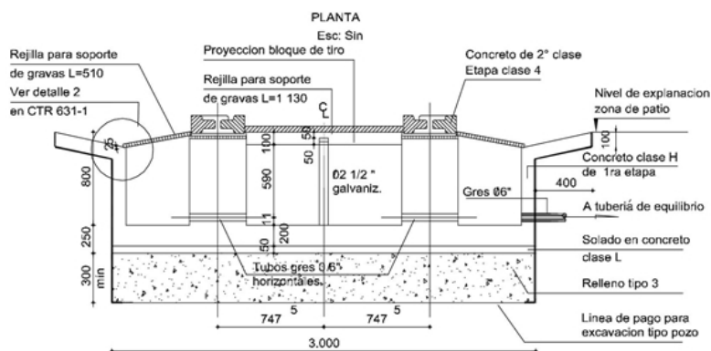
CORTE A-A Esc: Sin
