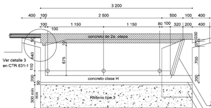
CORTE B-B Esc: Sin
