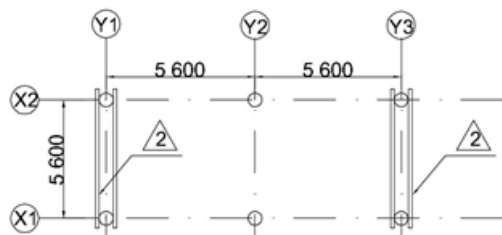
AISLADOR DE ESPIGO NIVEL ③ 5,80 m. Esc.: Sin
