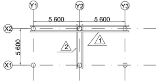
VIGA DE CIERRE NIVEL ⑨ 8,80 m NIVEL ⑩ 9,00 m Esc.: Sin
