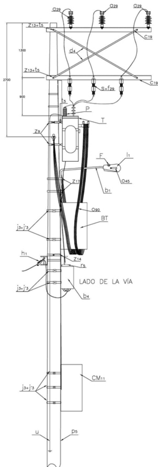
VISTA PERFIL
