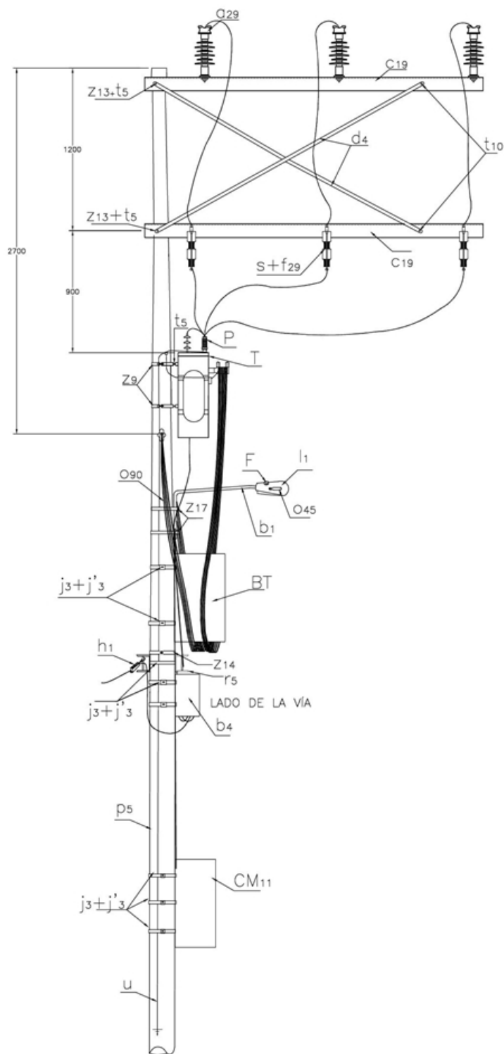
VISTA PERFIL
