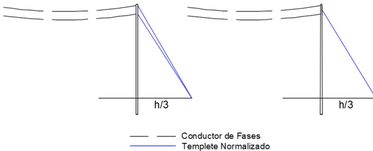
Figura 3. Disposición para la instalación de templete
