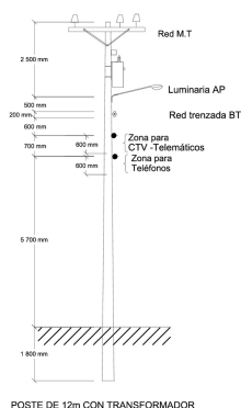
POSTE DE 12m CON TRANSFORMADOR
