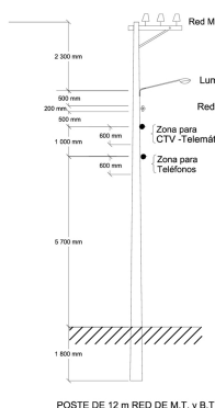
POSTE DE 12 m RED DE M.T. y B.T
