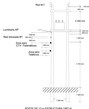
POSTE DE 12 m ESTRUCTURA TIPO H
