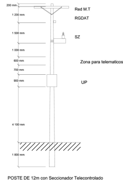
POSTE DE 12m con Seccionador Telecontrolado
