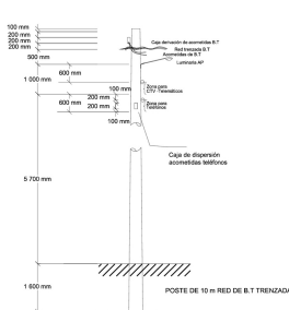
POSTE DE 10 m RED DE B.T TRENZADA
