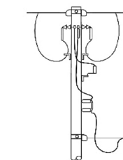
DERIVACIÓN A AISLADO CON SECCIONAMIENTO (LA 682-1)
