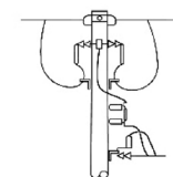
DERIVACIÓN A DESNUDO CON SECCIONAMIENTO (LA 679-1)
