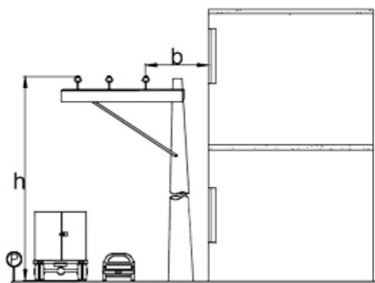
Fig. 5 DISTANCIA HORIZONTAL ENTRE CONDUCTORES Y VENTANAS O BALCONES DE EDIFICACIONES. DISTANCIA VERTICAL EN PARQUEADEROS
