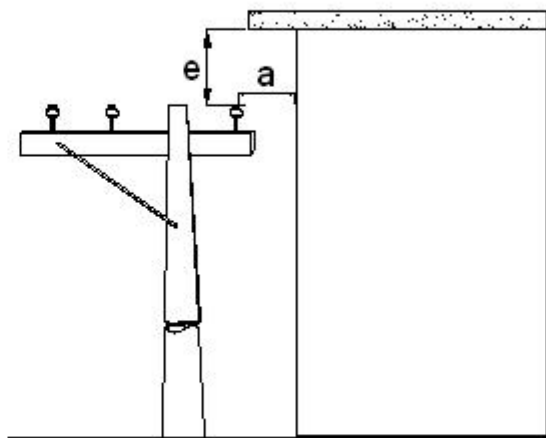
Fig. 2 DISTANCIA HORIZONTAL ENTRE CONDUCTORES Y PAREDES DE EDIFICACIONES
