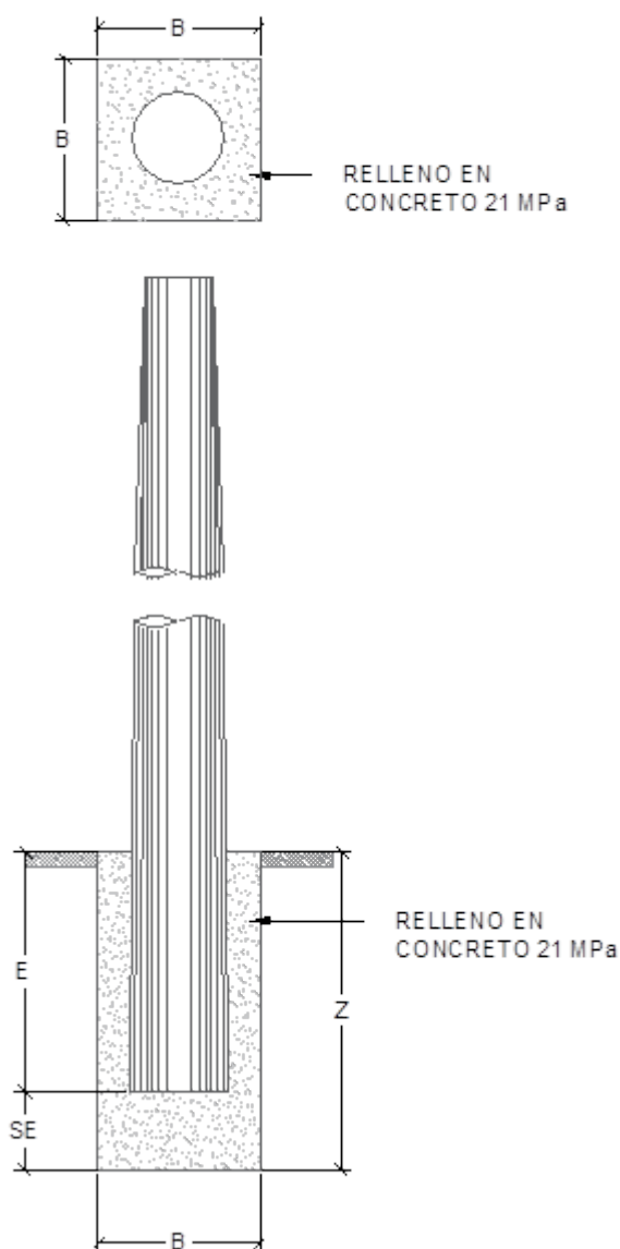
Figura 3 cimentación ccuadrada relleno en concreto
