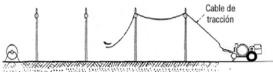
Figura 5c. Tendido cuerda de tiro
