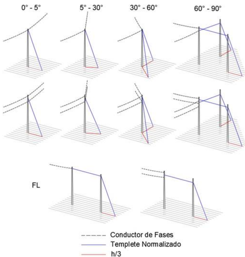
Figura 3. Disposición para la instalación de templates
