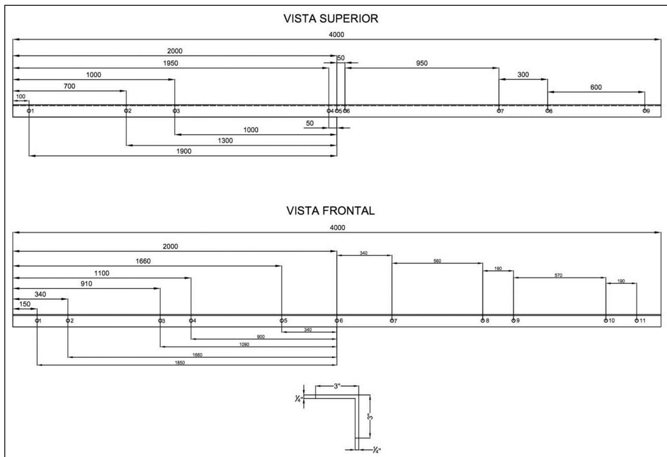
Figura 2. Cruceta metálica de 4 m.
