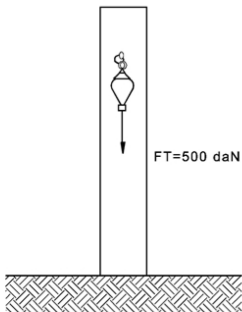
FIG. 4 ENSAYO DE TRACCIÓN
