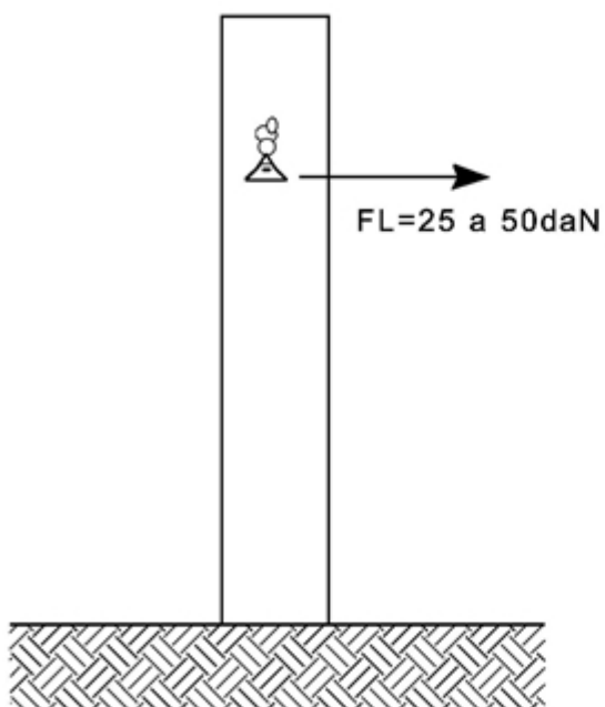
FIG. 3 ENSAYO DE DESLIZAMIENTO
