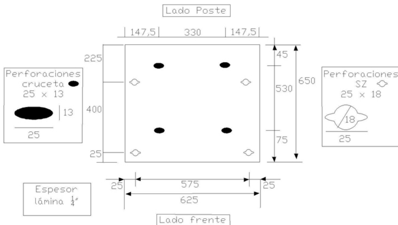
Figura 2. Base Seccionador bajo carga telecontrolado marca ICET para instalar en bandera.
