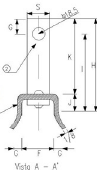
FIGURA 2. DIMENSIONES Y COMPONENTES PARA AISLADOR DE UN SOLO PUESTO
