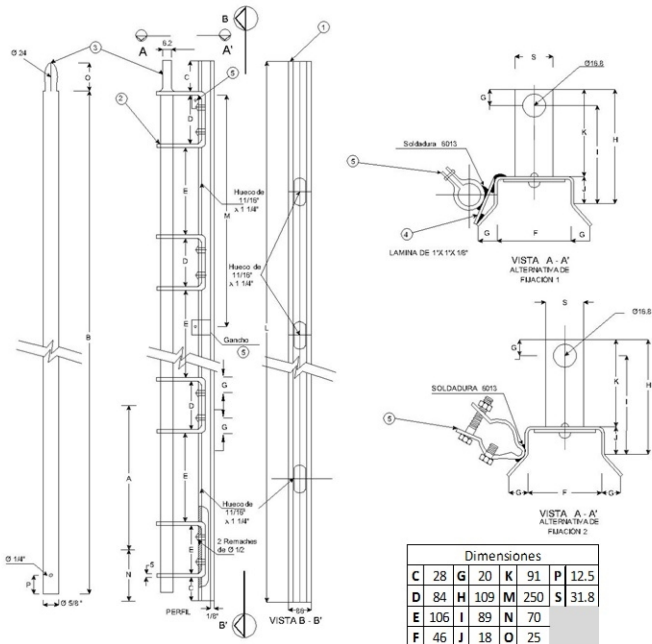
FIGURA 1. DIMENSIONES Y COMPONENTES
