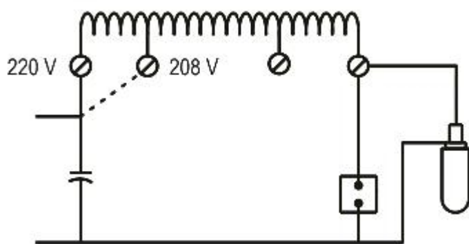
Arrancador tipo Impulsador paralelo
