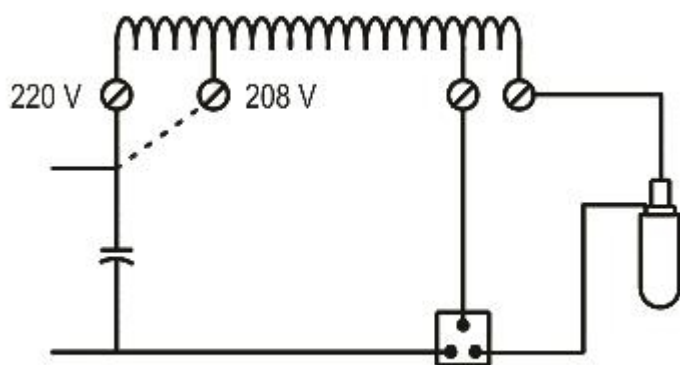
Arrancador tipo Impulsador de derivación
