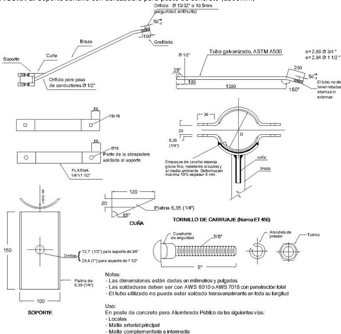
FIGURA 1. Soporte sencillo con abrazadera para poste de concreto (1500mm)
