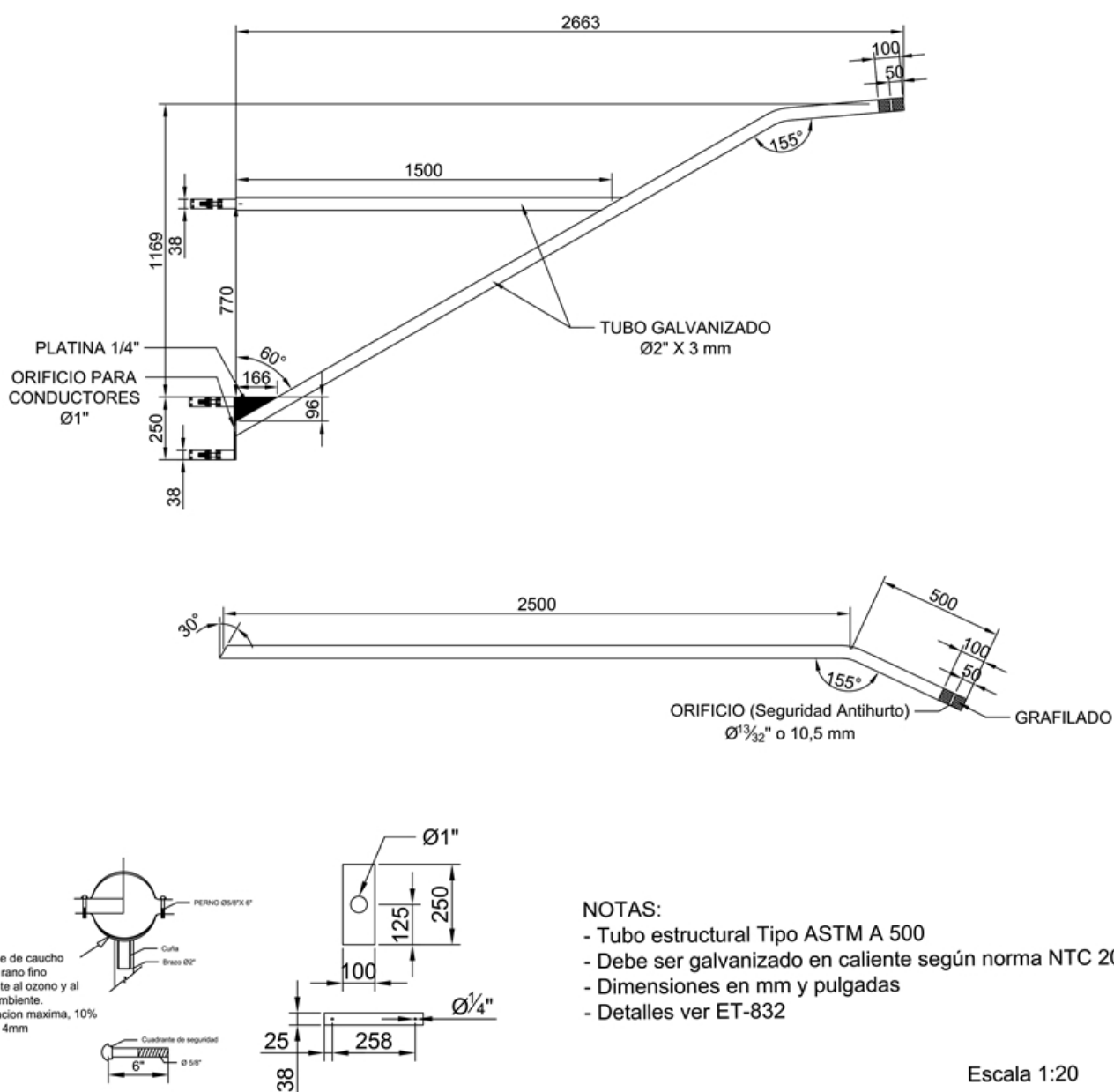
FIGURA 14A. Soporte extendido doble tubo para luminaria horizontal con abrazadera (Alternativa 4 - 2663mm)
