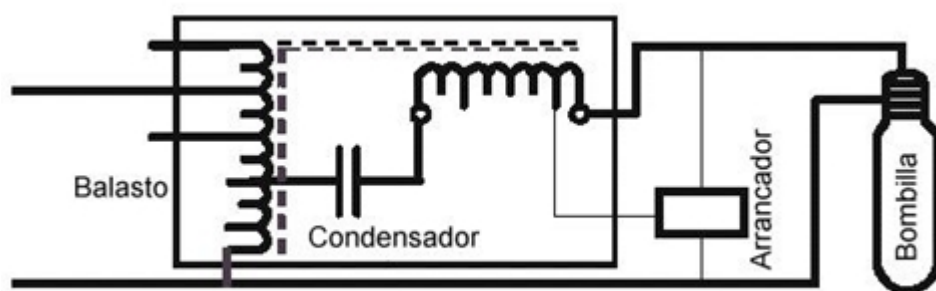
Figura 2: Diagrama de conexión balasto CWA
