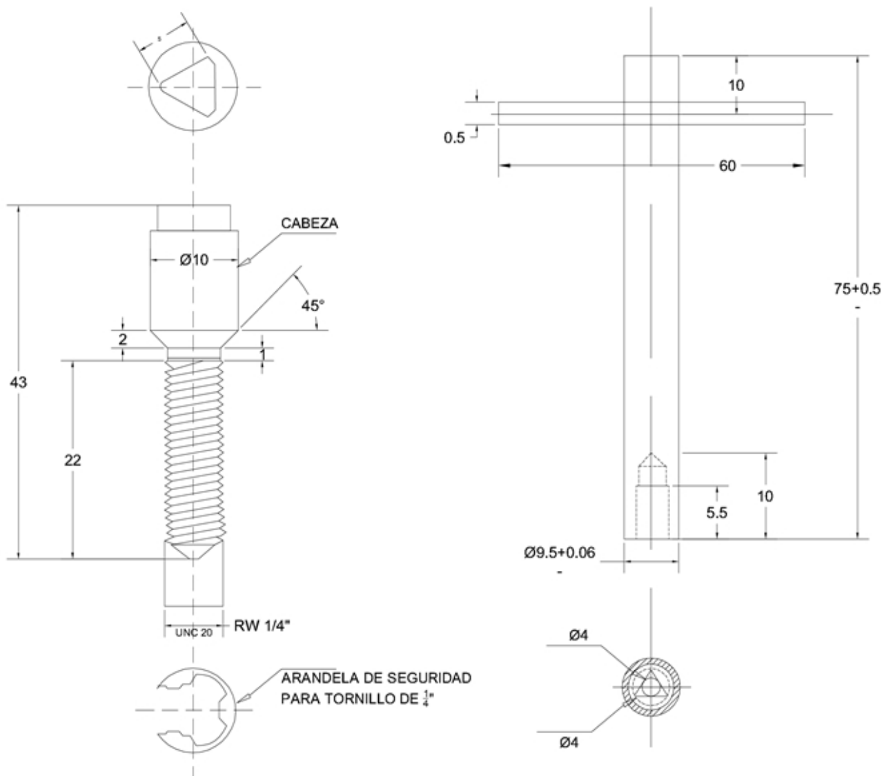
Figura 3. Tornillo y llave de seguridad
