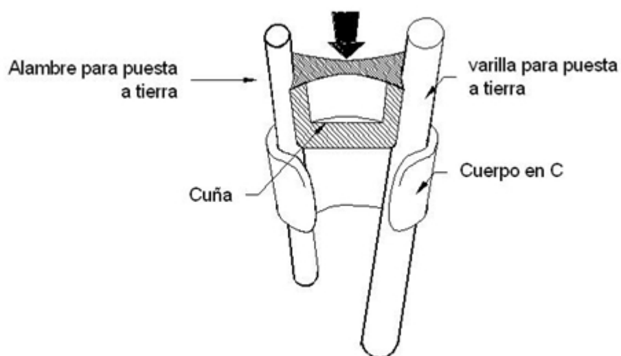
FIGURA 2. CONECTOR DE PUESTA A TIERRA DEL TIPO CUÑA
