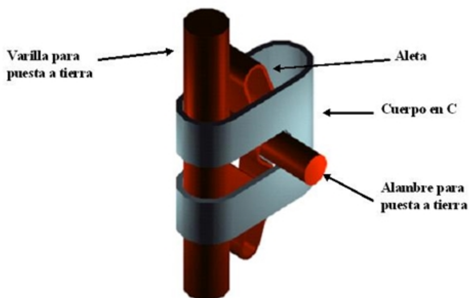
FIGURA 1. CONECTOR DE PUESTA A TIERRA DEL TIPO CUÑA TRANSVERSAL
