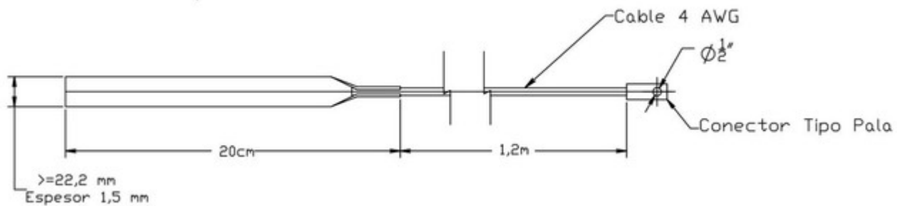
Figura 7. Acople fleje a terminal \frac{1}{2} ".
