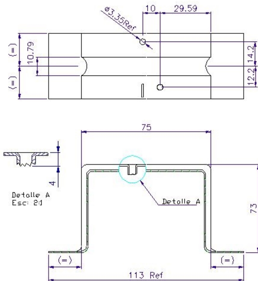
FIGURA 9. SOPORTE INTERRUPTOR
