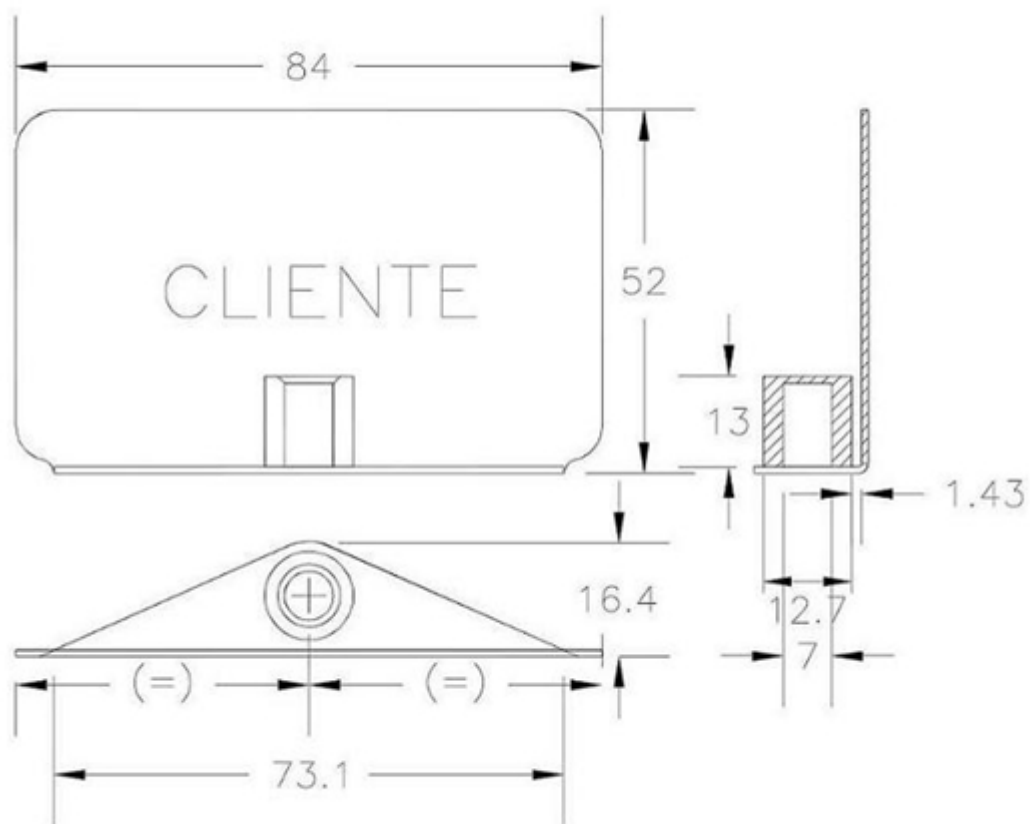
Figura 11. TAPA CORREDIZA
