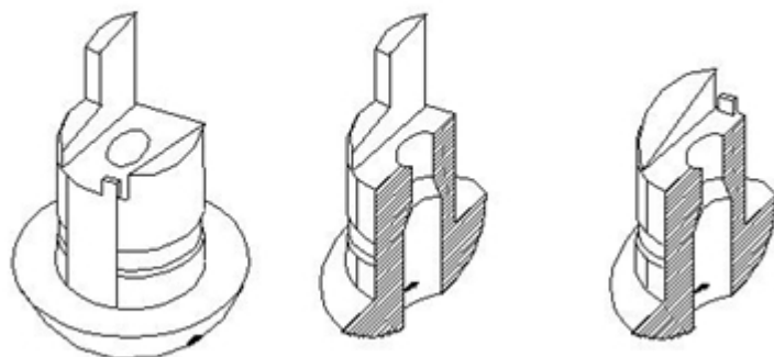
PERSPECTIVA DEL BUJE (NORMA ET 905 - 9A)
