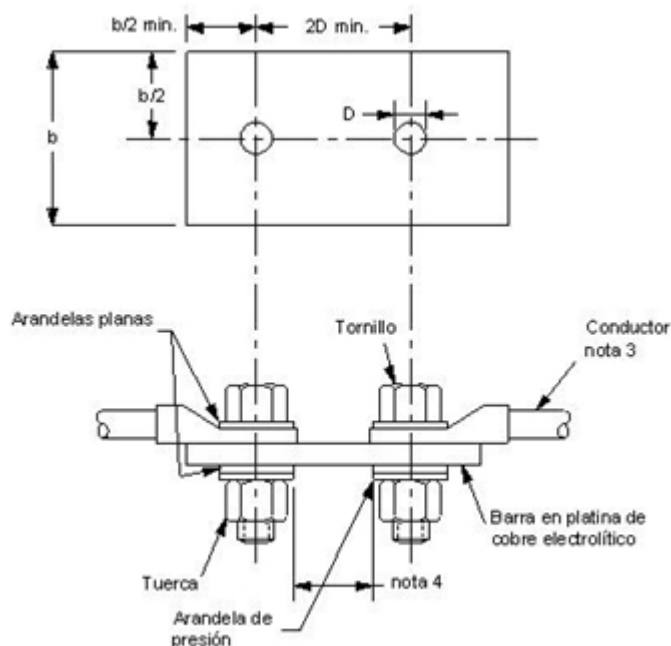
FIGURA 3. FIJACIÓN DE LAS DERIVACIONES DEL BARRAJE
