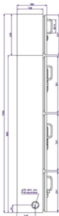
FIGURA 3: VISTA LATERAL
