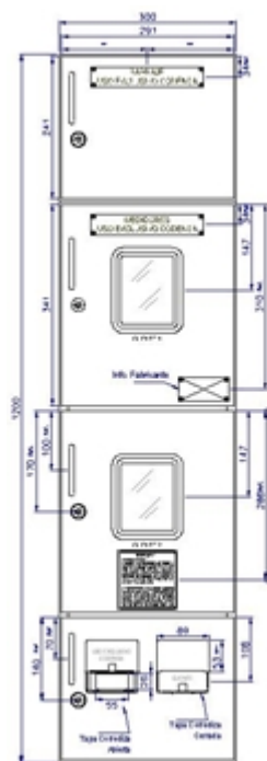
FIGURA 1. VISTA FRONTAL
