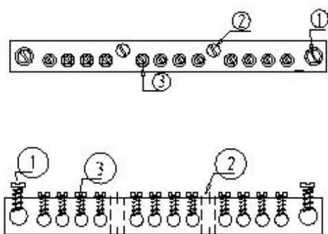
FIGURA 4. DETALLE DE BORNERAS DE FASE Y NEUTRO
