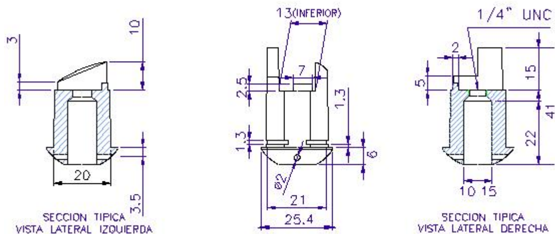
FIGURA 9. BUJE DEL SISTEMA DE SEGURIDAD
