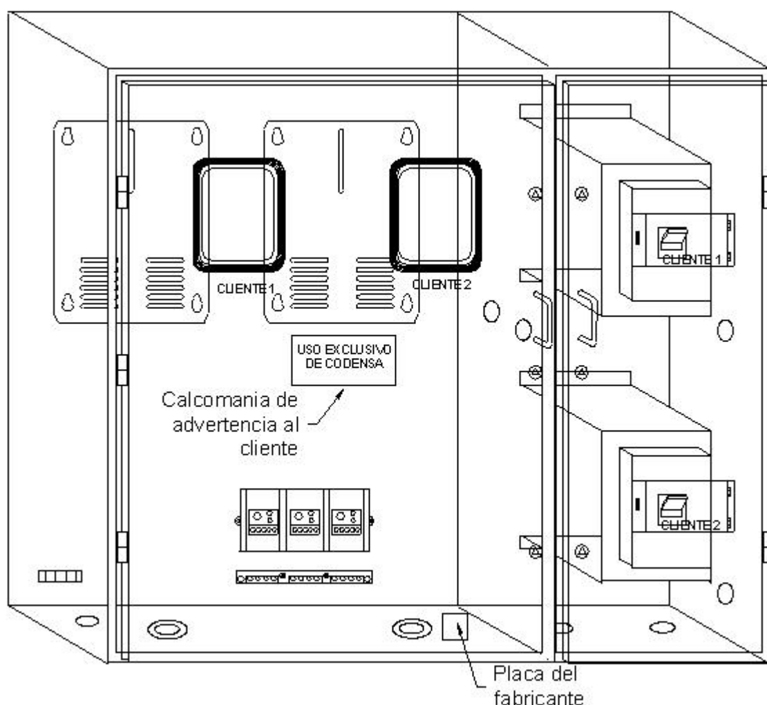
FIGURA 1 (VISTA ISOMETRICA)
