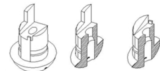
FIGURA 9B. BUJE DE SEGURIDAD
