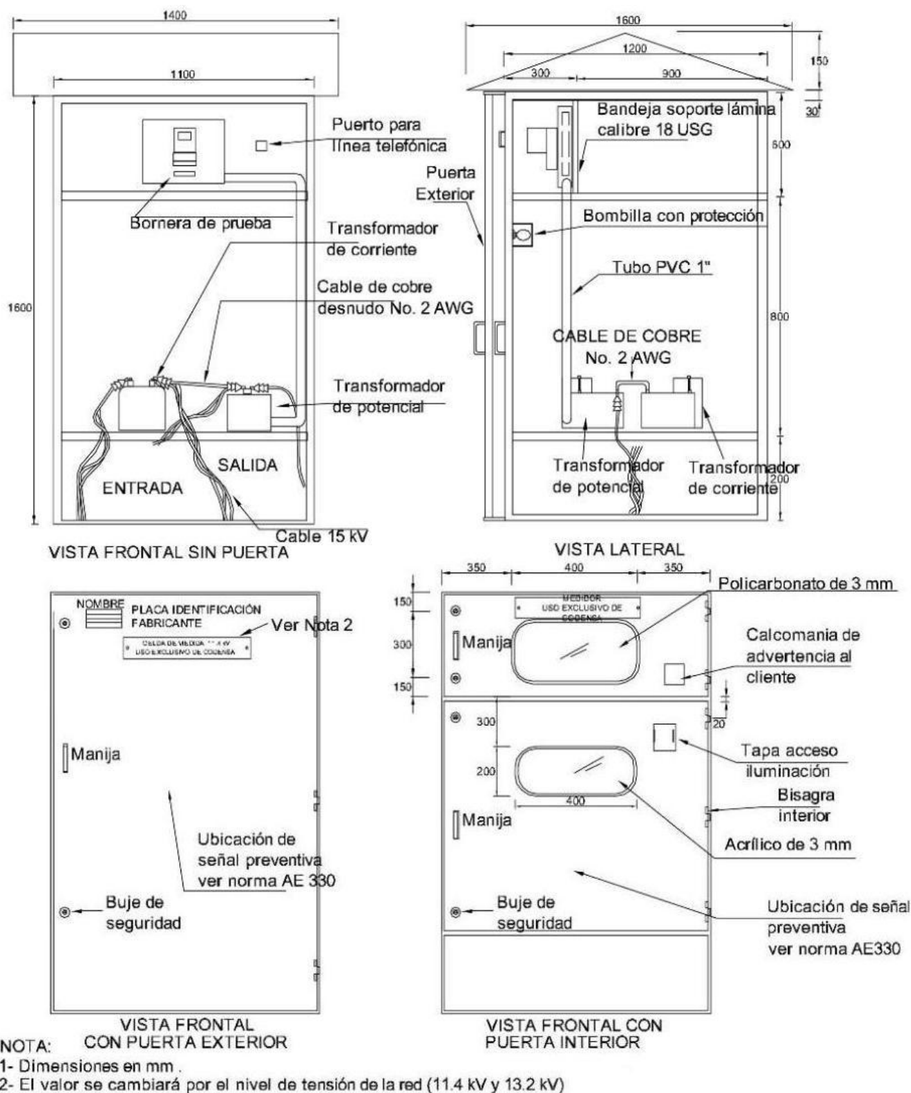
FIGURA 8. CELDA DE MEDIDA 34,5kV TIPO INTEMPERIE
