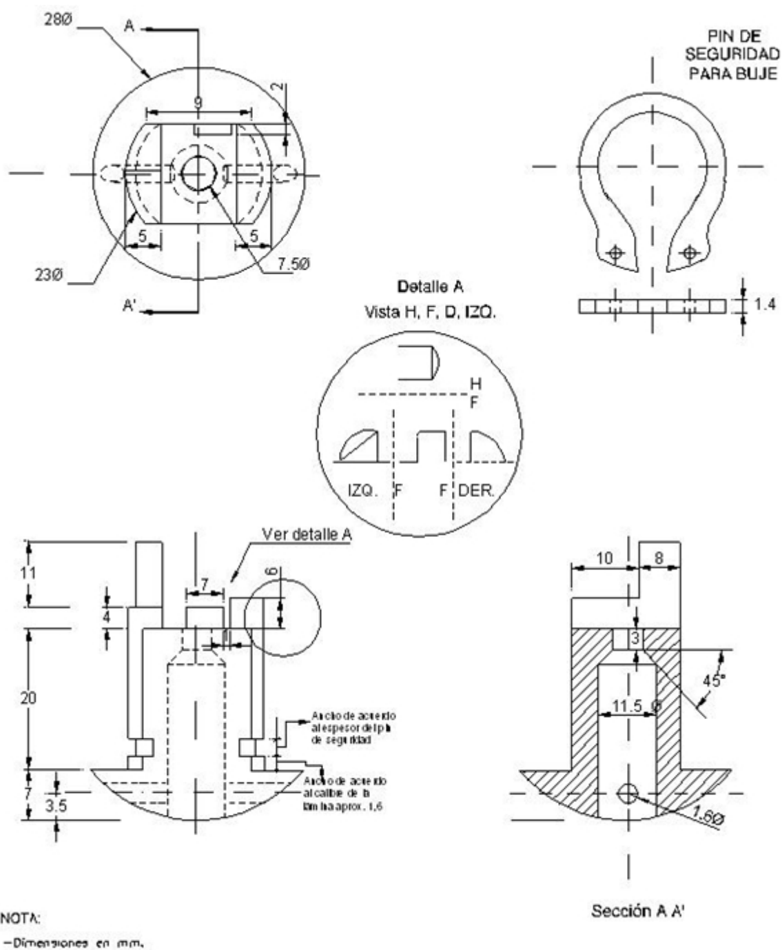
FIGURA 10. BUJE DE SEGURIDAD
