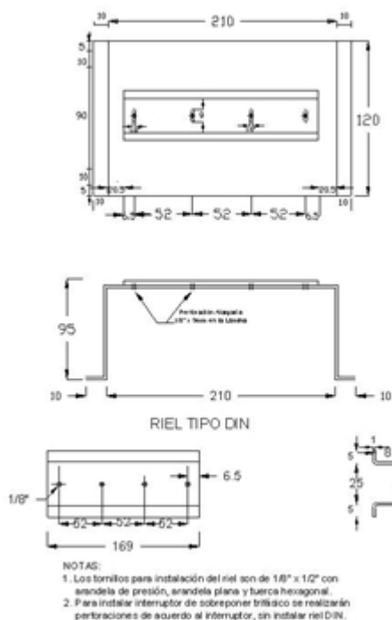
FIG 5 SOPORTE PARA INTERRUPTORES TERMOMAGNÉTICOS
