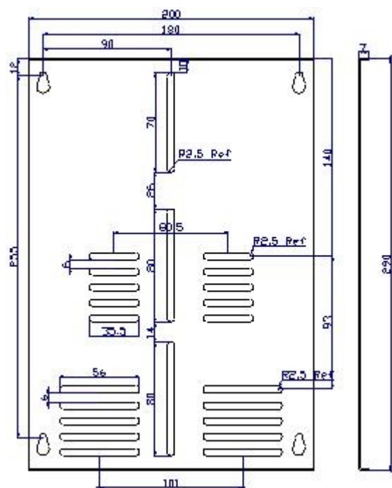
fig 10 BANDEJA PARA MEDIDOR MONOFÁSICO / TRIFÁSICO
