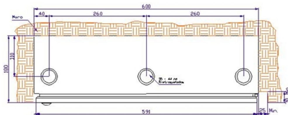
FIGURA 5. VISTA SUPERIOR
