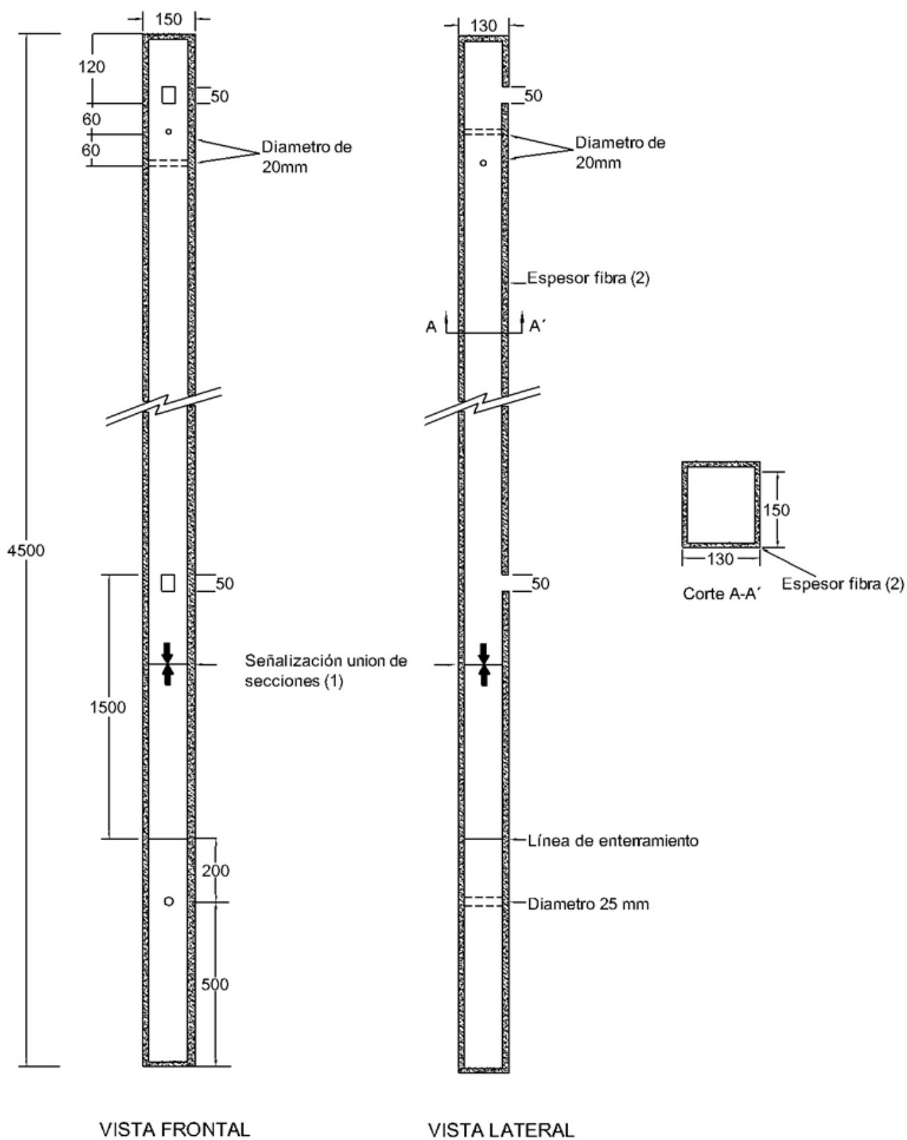
FIGURA 1. ESQUEMA POSTE EN FIBRA
