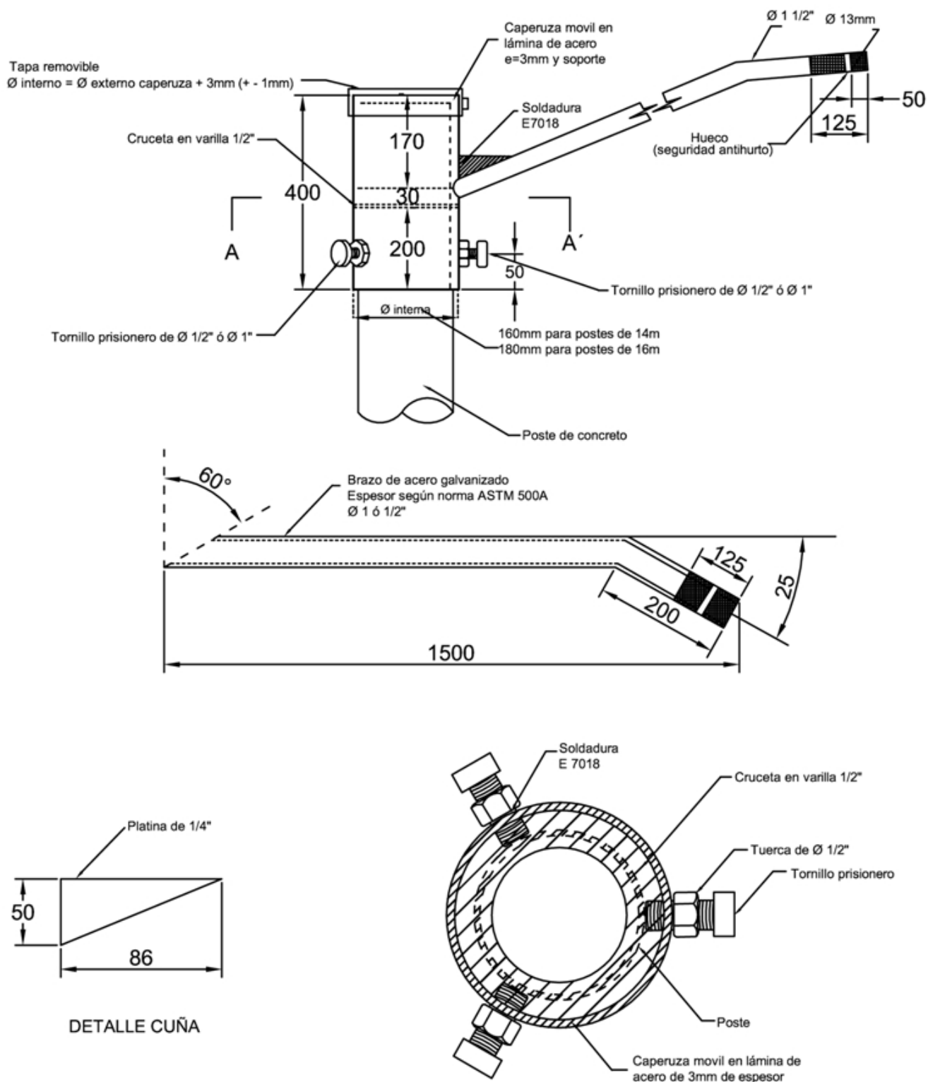
FIGURA 5. Soporte sencillo para luminaria
