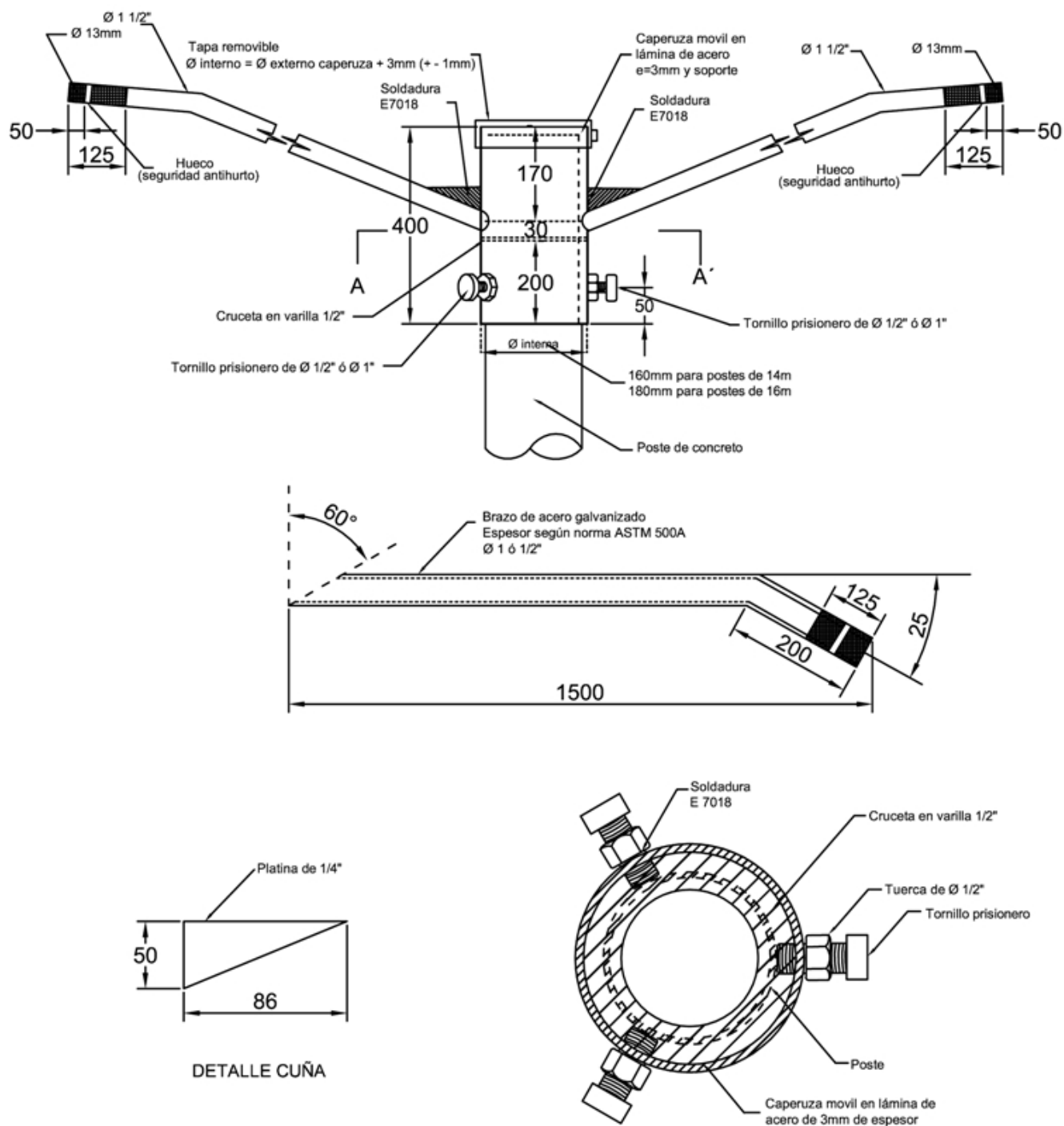
FIGURA 6. Soporte doble para luminaria
