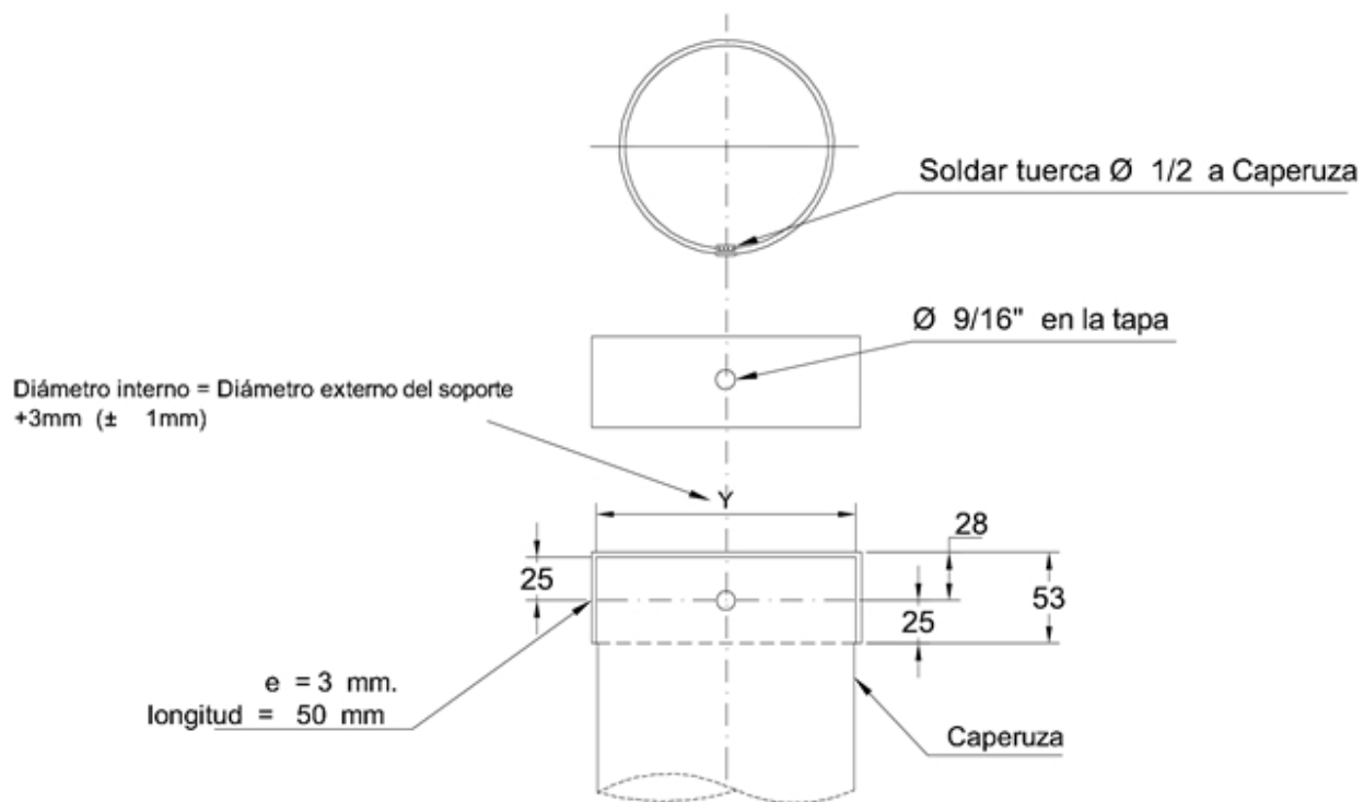
FIGURA 7. Detalle de la tapa removible.
