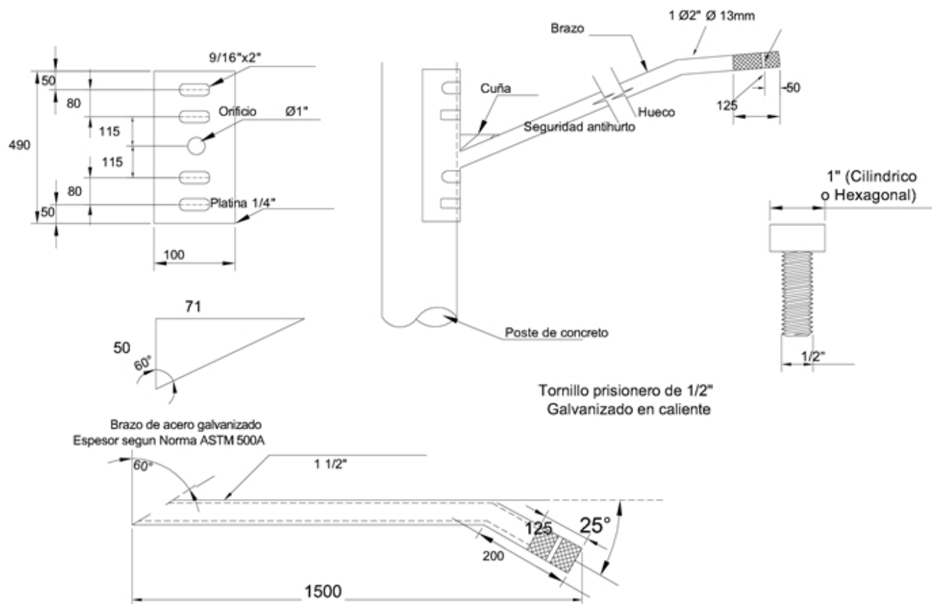
FIGURA 8. Soporte para luminaria peatonal 9000 mm.
