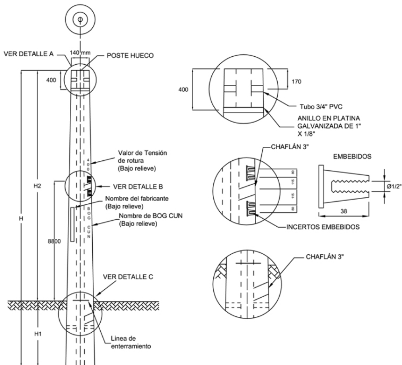
FIGURA 1. Dimensiones de poste esbelto
